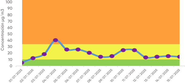
Ozono (O 3 )
